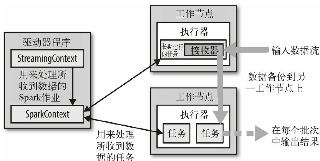
图 10-5: Spark Streaming 在 Spark 各组件中的执行过程
