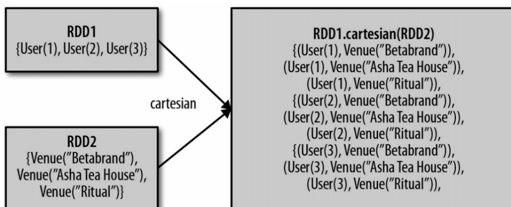
图 3-5: 两个 RDD 的笛卡儿积
