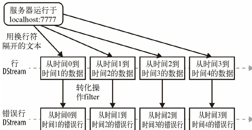
图 10-3: 例 10-4 至例 10-8 中的 DStream 及其转化关系
