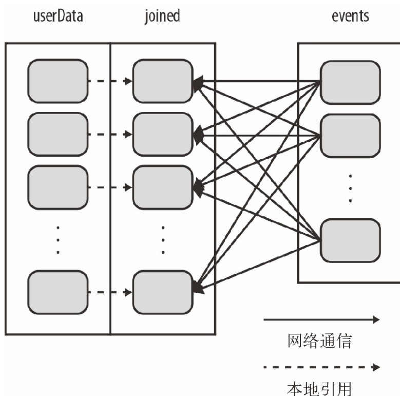
图 4-5: 使用 partitionBy() 时对 userData 和 events 进行连接操作
