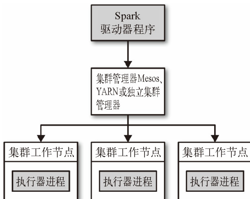
图 7-1: 分布式 Spark 应用中的组件
