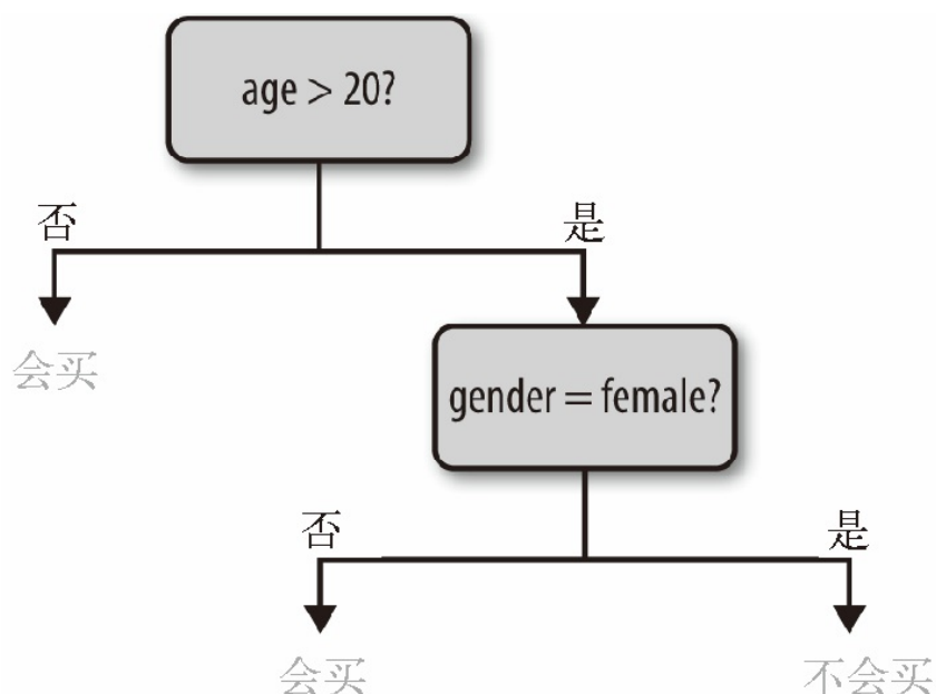
图 11-2: 一个预测用户是否会购买一件产品的决策树示例
