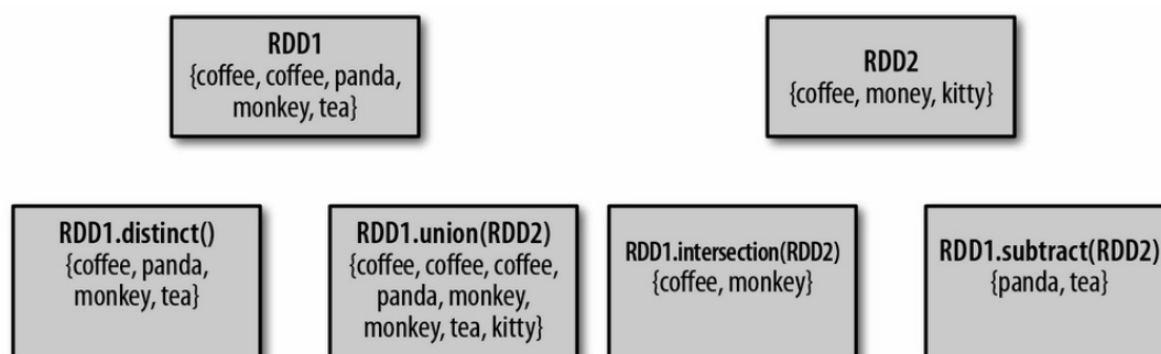
图 3-4: 一些简单的集合操作
