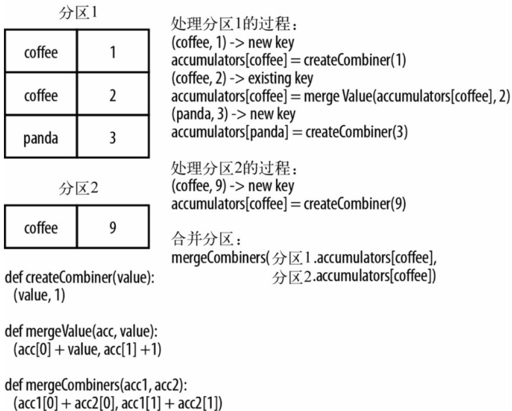
图 4-3: combineByKey() 数据流示意图
