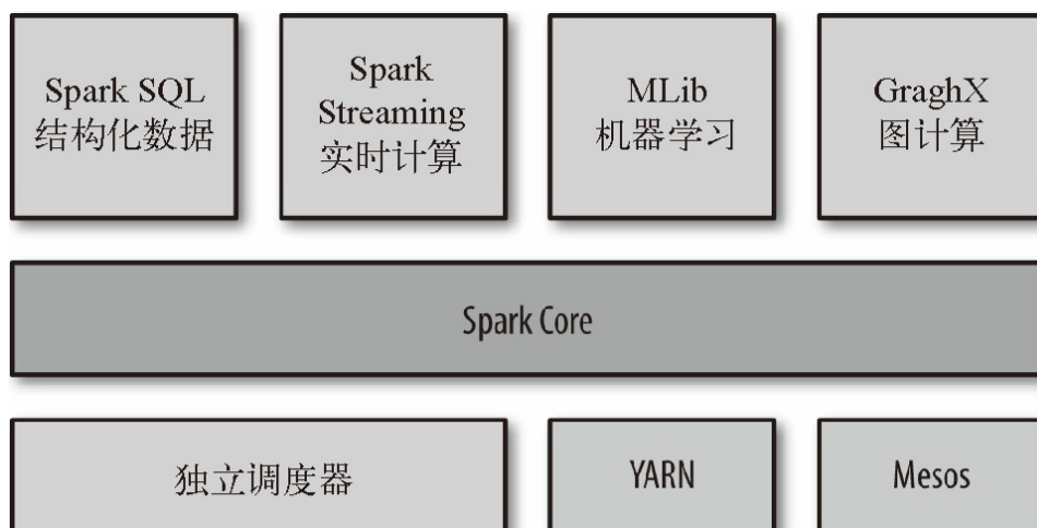
图 1-1: Spark 软件栈
