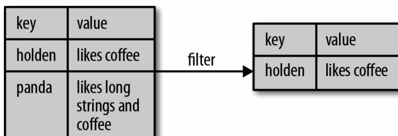
图 4-1：根据值筛选
