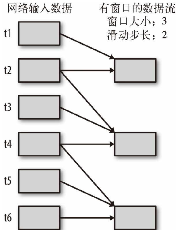
图 10-6: 一个基于窗口的流数据，窗口时长为 3 个批次，滑动步长为 2 个批次；每隔 2 个批次就对
