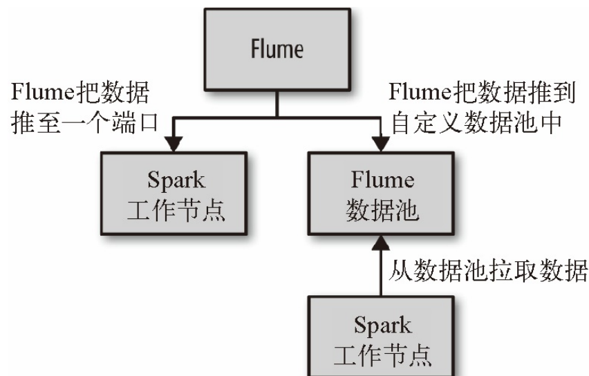
图 10-8: Flume 接收器选项
