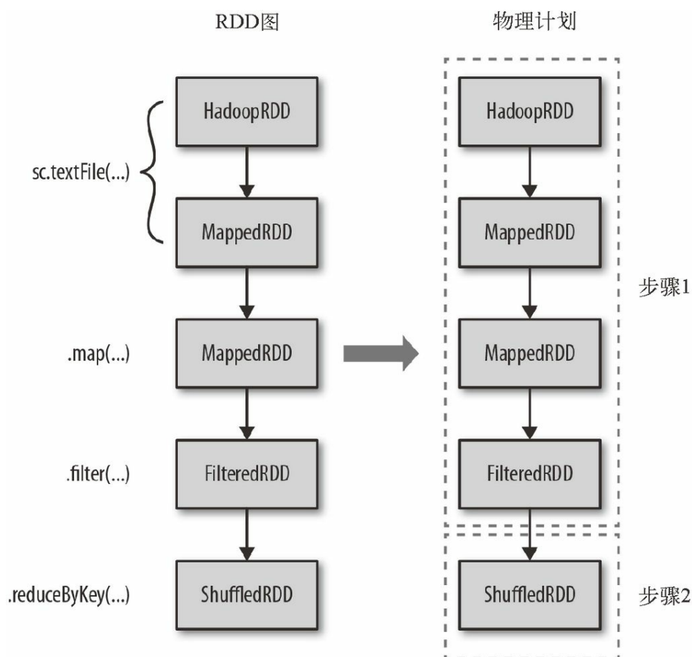
图 8-1: 将 RDD 转化操作串联成物理执行步骤
