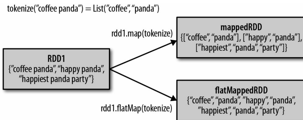
图 3-3: RDD 的 flatMap() 和 map() 的区别
