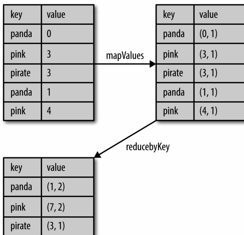
图 4-2: 求每个键平均值的数据流
