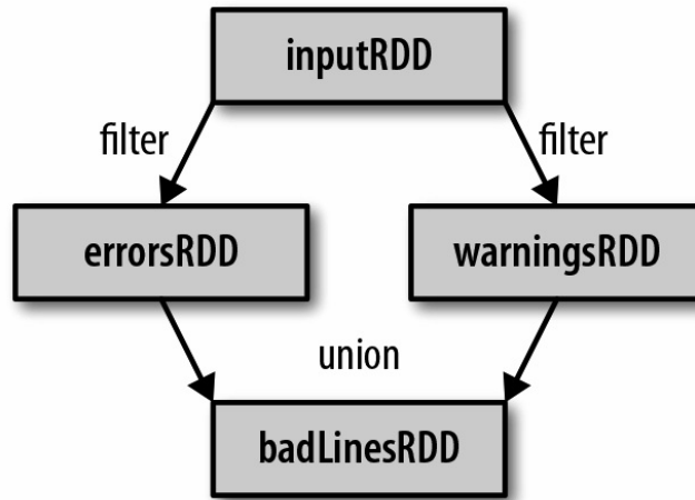
图 3-1: 日志分析过程中创建出的 RDD 谱系图
