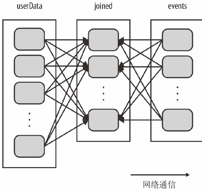
图 4-4: 未使用 partitionBy() 时对 userData 和 events 进行连接操作
