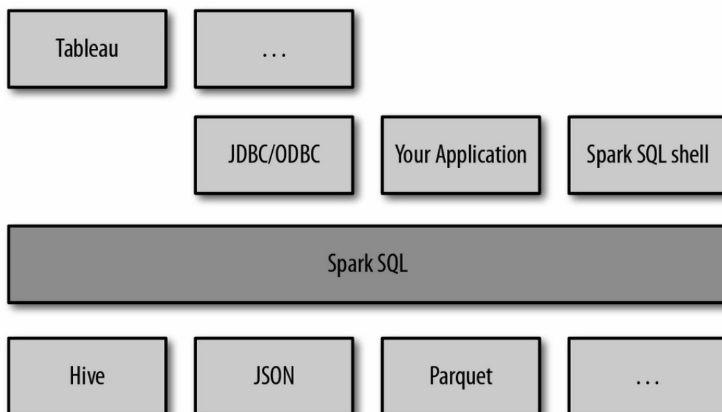
图 9-1: Spark SQL 的用途
