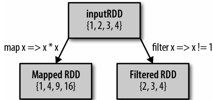
图 3-2: 从输入 RDD 映射与筛选得到的 RDD
