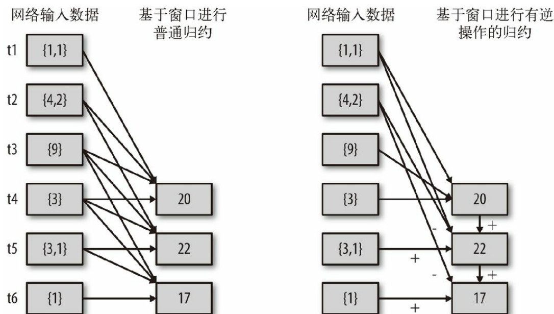
图 10-7: 普通的 reduceByWindow() 与使用逆函数的增量式 reduceByWindow() 的区别
