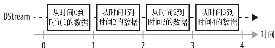
图 10-2: DStream 是一个持续的 RDD 序列
