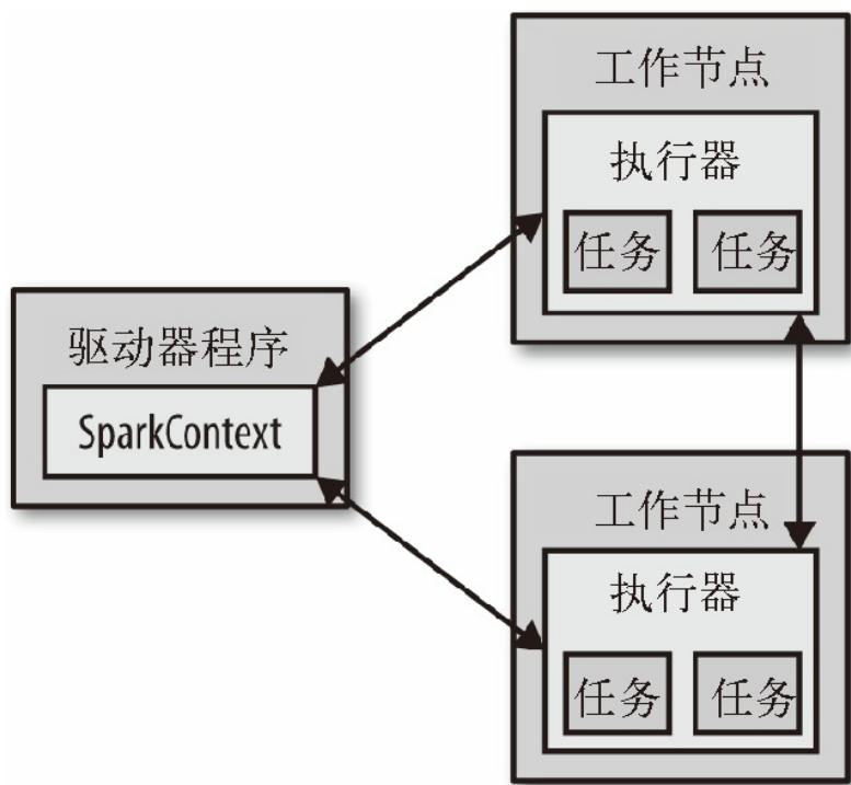
图 2-3: Spark 分布式执行涉及的组件
