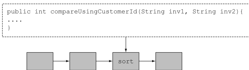
图1-3 将compareUsingCustomerId方法作为参数传给sort
