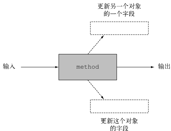
图13-2 带有副作用的函数
