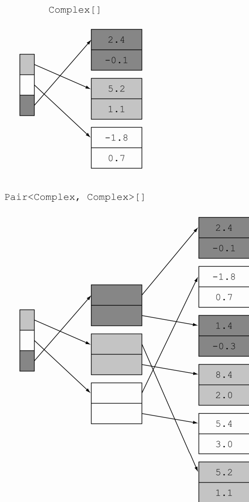
图16-1 对象与值类型
