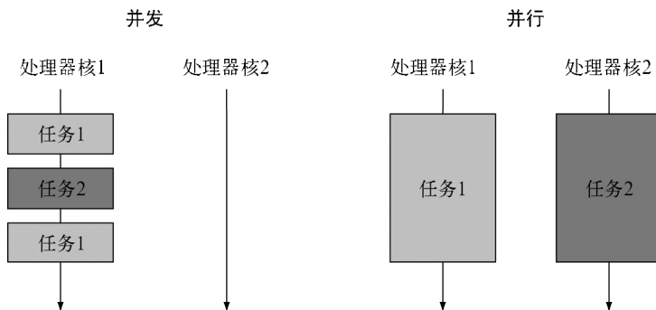
图11-2 并发和并行
