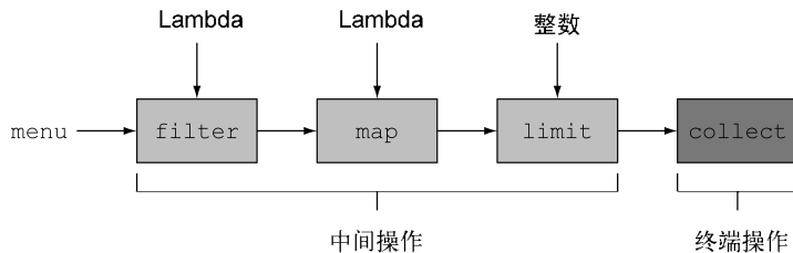
图4-5 中间操作与终端操作
