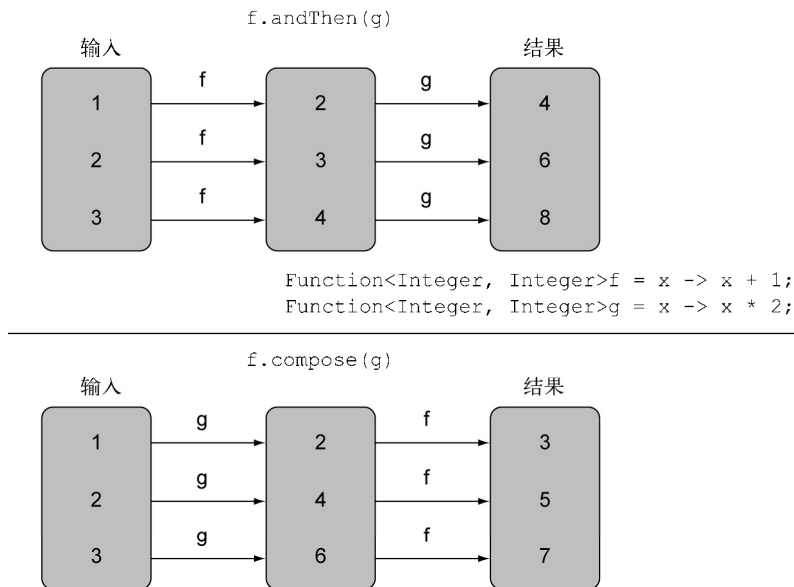
图3-6 使用andThen与compose
