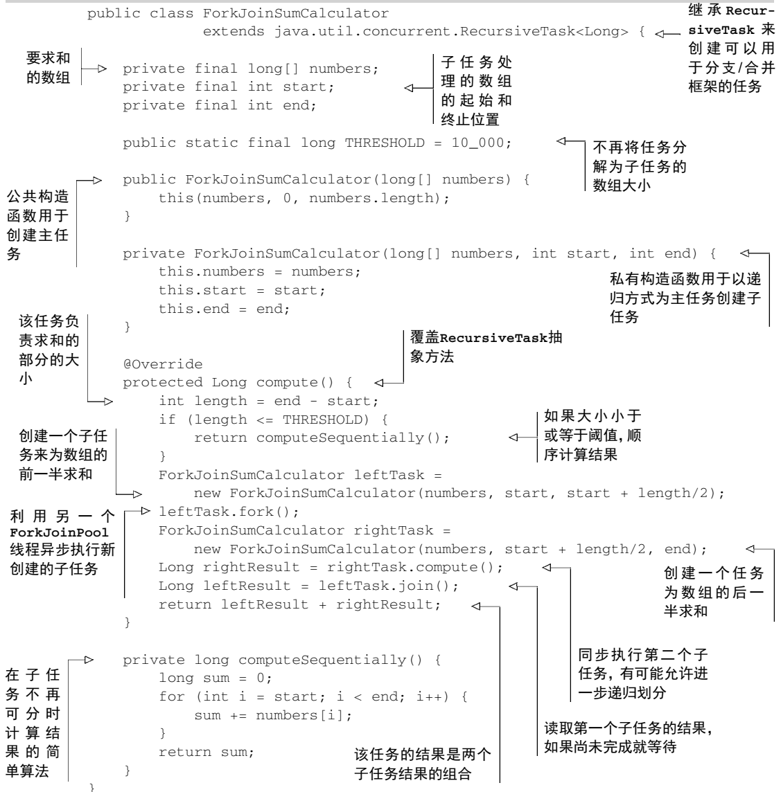
代码清单7-2 用分支/合并框架执行并行求和
