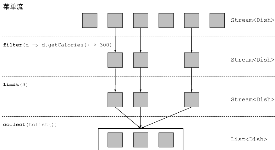
图5-3 截短流
