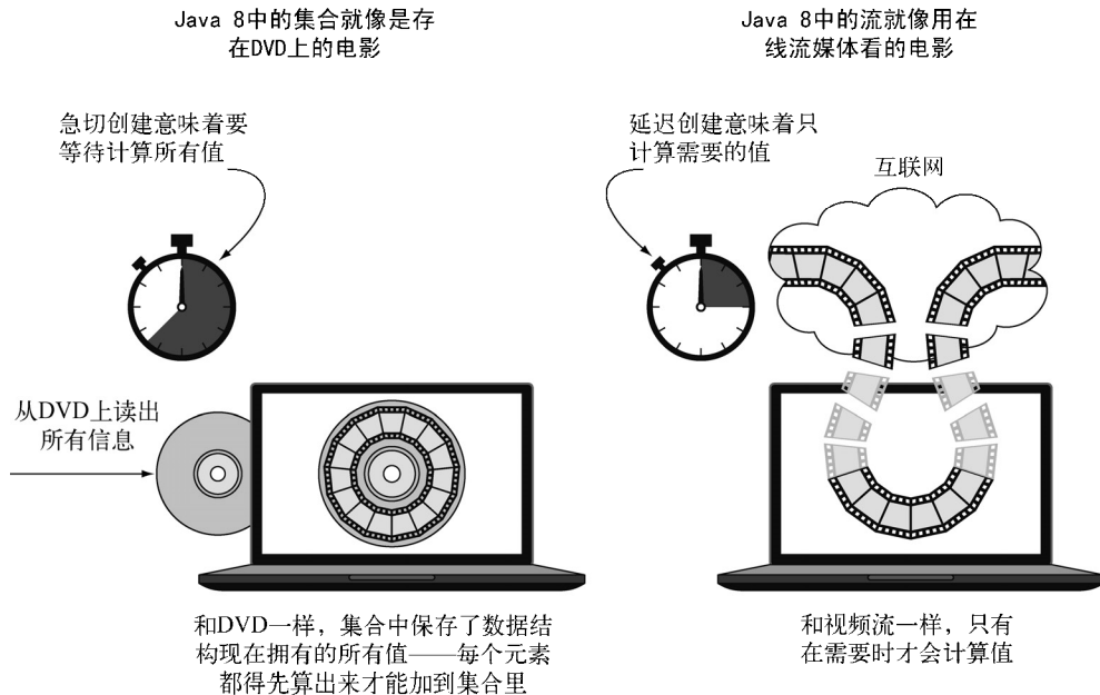
图4-3 流与集合
