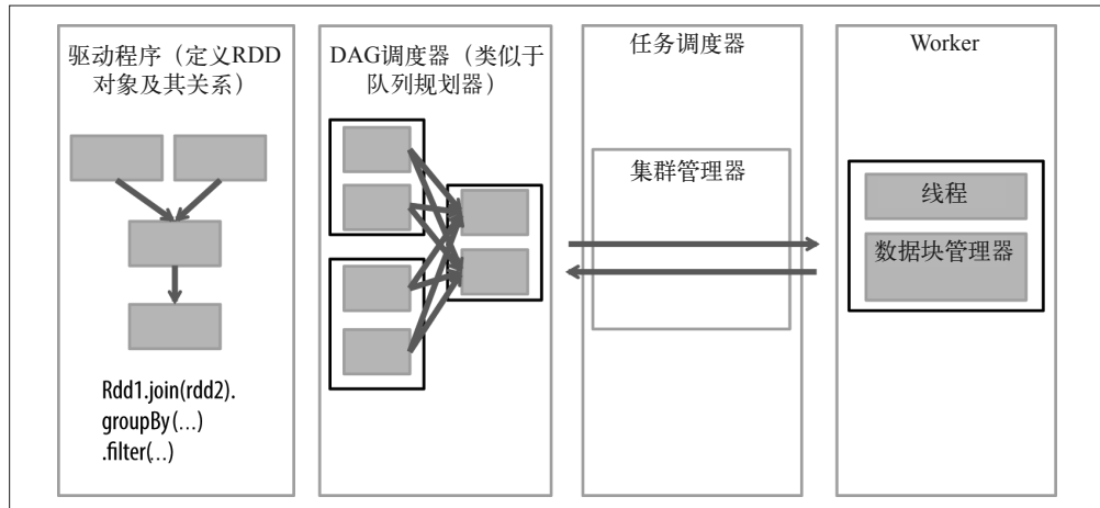
图 3-6: Spark 组件
