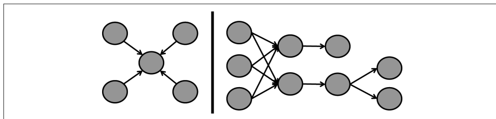
图 3-5: 有向无环图
