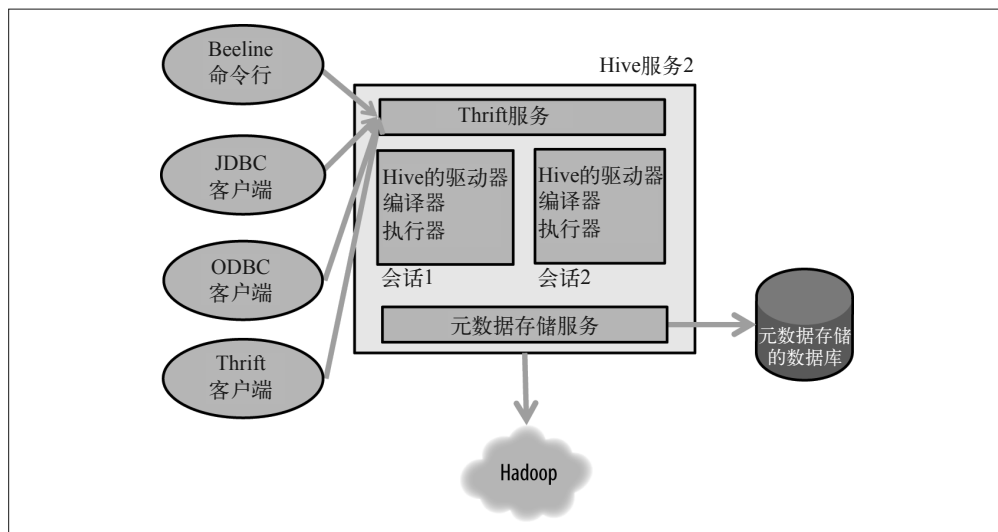
图 3-10: Hive 的架构
